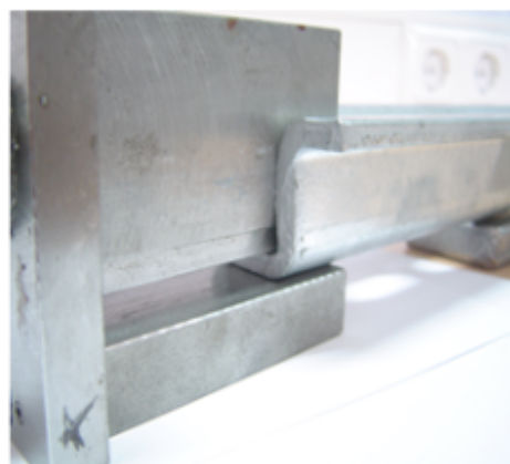
Bild Nr.2. Ansetzen der Prüflehre.
