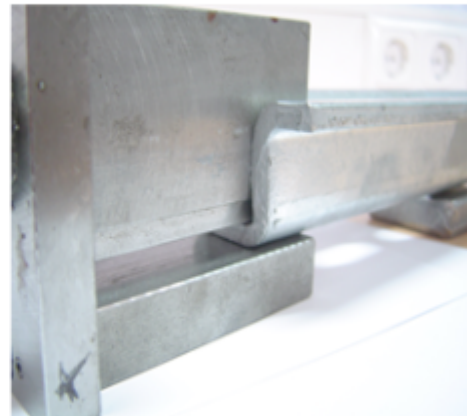
Bild Nr.2. Ansetzen der Prüflehre.
