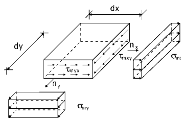
Bild 1.2 — Membranspannungen
