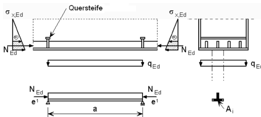
Bild 5.2 — Definition der Querschnittsfläche A_i
