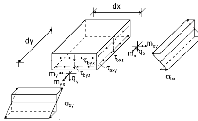
Bild 1.3 — Längs- und Schubspannungen infolge Biegung
