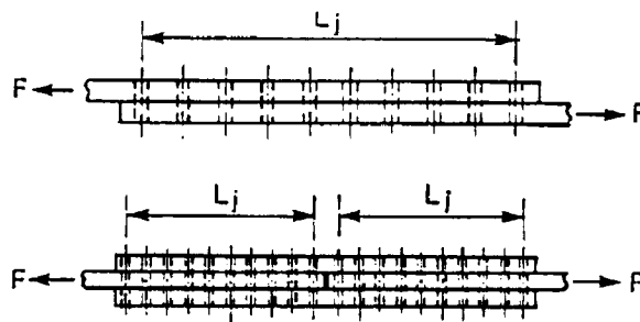
Bild 3.7 — Lange Anschlüsse
