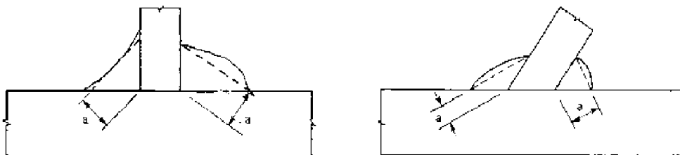
Bild 4.3 — Kehlnahtdicke
