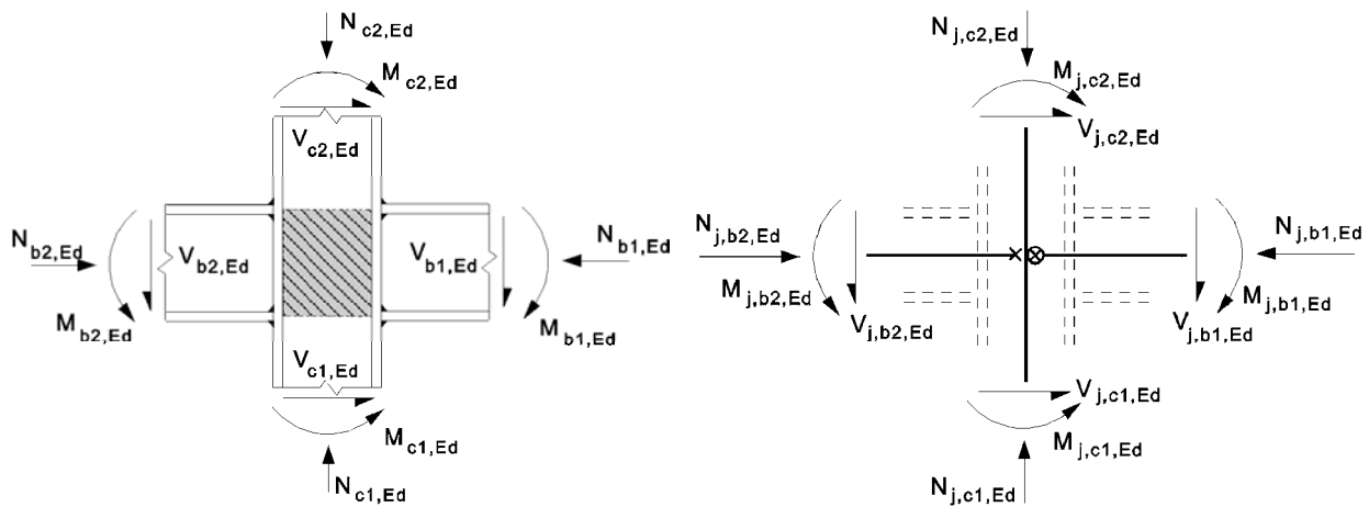
a) Werte am Anschnitt des Stegfeldes
