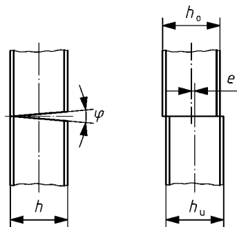
Bild NA.1 — mögliche Ausführungen von Kontaktstößen (a) Teilkontakt, b) und c) vollständiger Kontakt)
