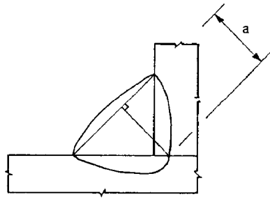
Bild 4.4 — Kehlernahtdicke bei tiefem Einbrand
