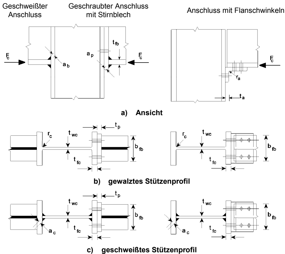
Bild 6.6 — Querdruk bei einer nichtausgesteiften Stütze
