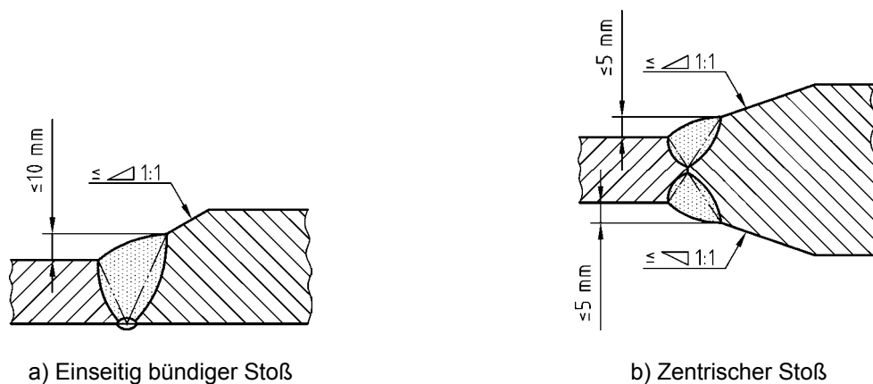
Bild NA.3 — Beispiele für das Brechen von Kanten bei Stumpfstoßen von Querschnittsteilen mit verschiedenen Dicken
