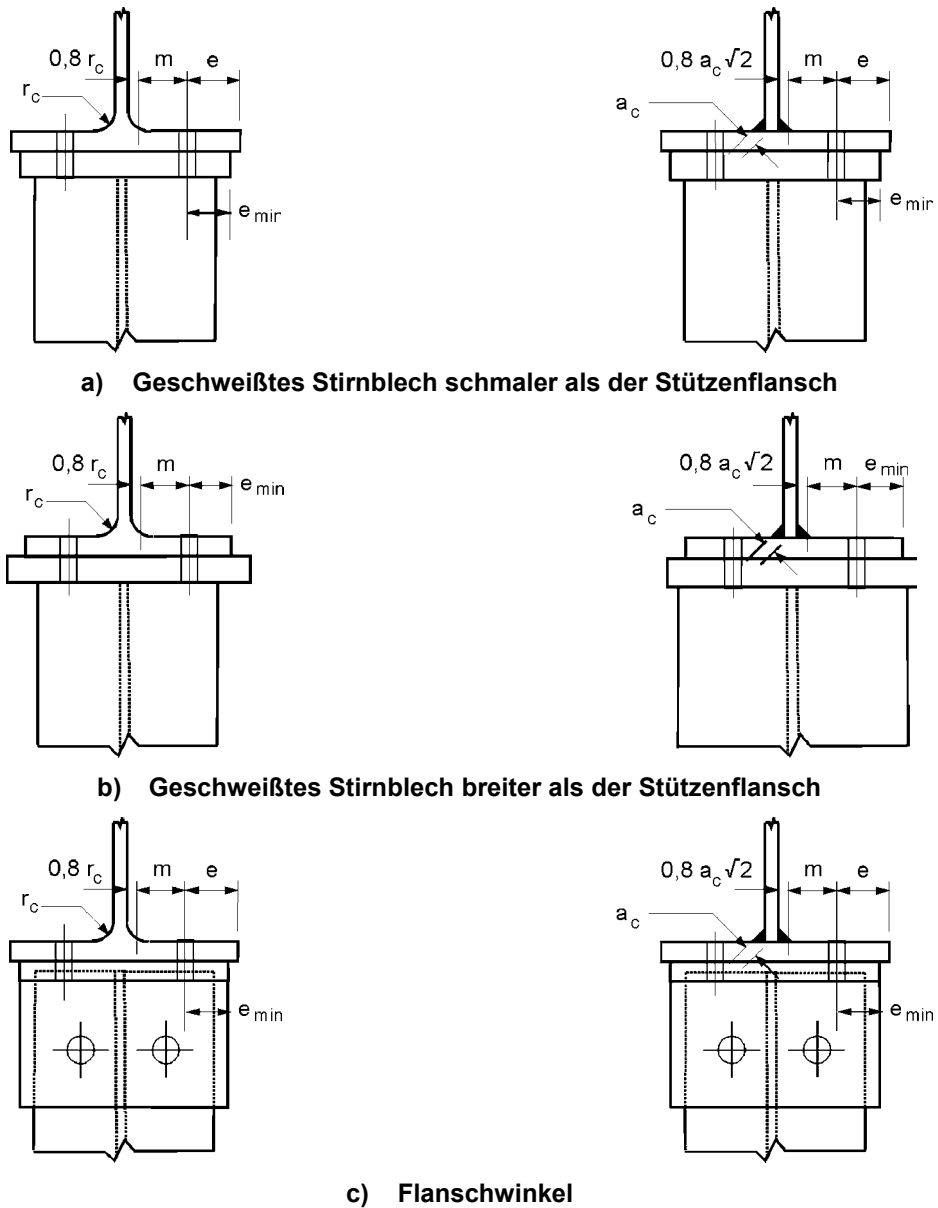
Bild 6.8 — Maße für e , e_{min} , r_c und m
