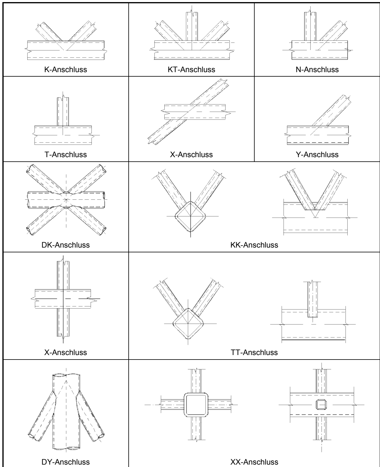
Bild 7.1 — Anschlussarten in Fachwerken mit Hohlprofilen
