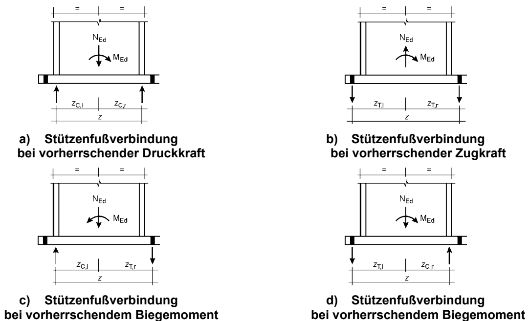
Bild 6.18 — Bestimmung des Hebelarms z bei Stützenfußverbindungen
