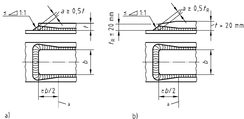
Bild NA.4 — Vorbinden zusätzlicher Gurtplatten
