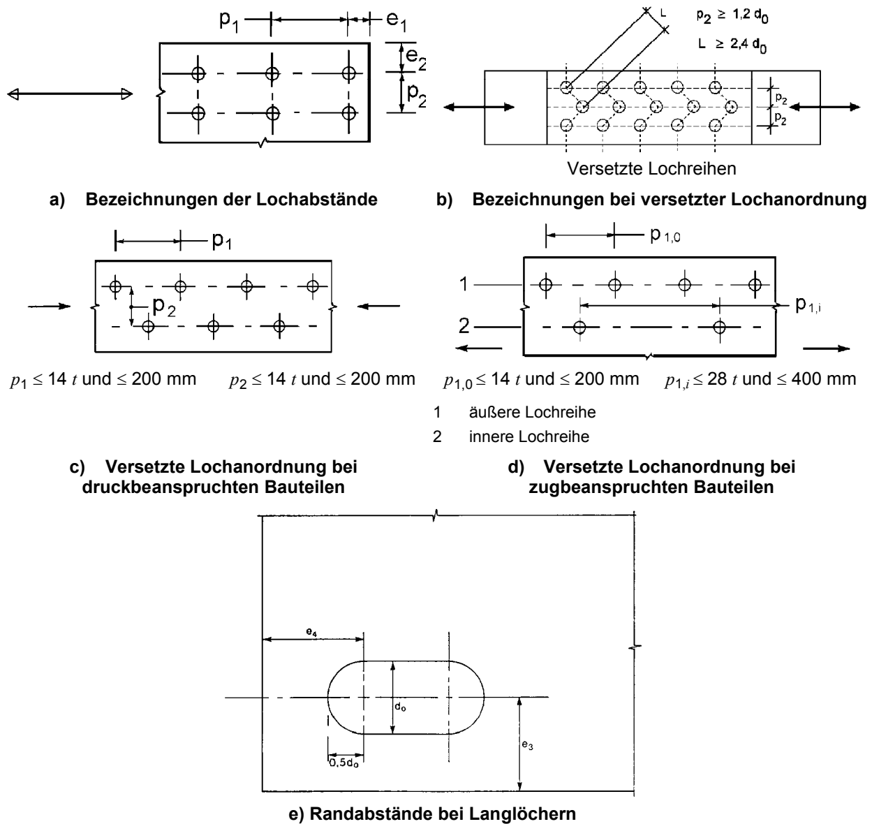
Bild 3.1 — Loch- und Randabstände von Verbindungsmitteln
