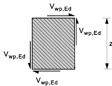
a) Schubkäfe im Stützenstegfeld
