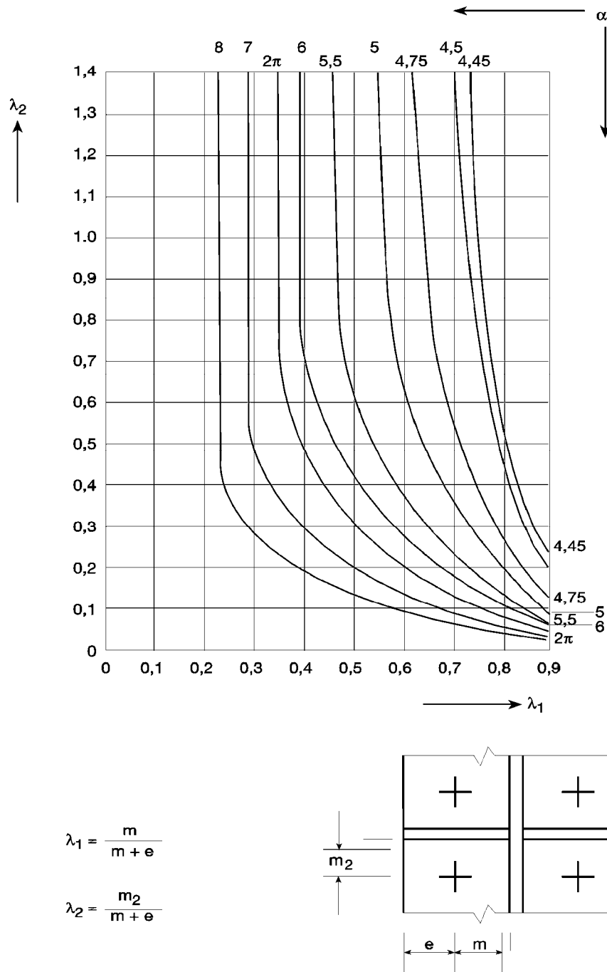
Bild 6.11 — \alpha -Werte für ausgesteifte Stützenflansche und Stirnbleche
