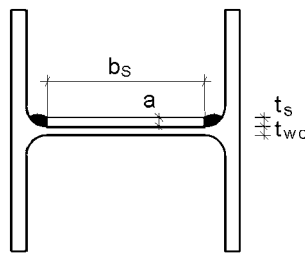
a) Anordnung
