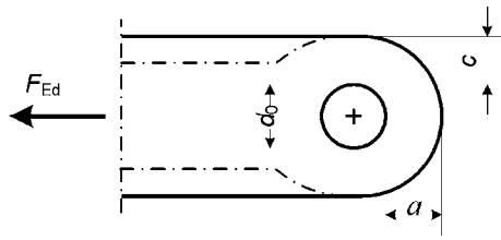
a) Lochdurchmesser und Dicke vorgegeben
