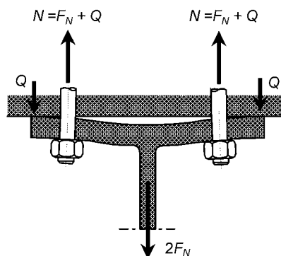
Bild 8.8 — Abstützkräfte (Q)
