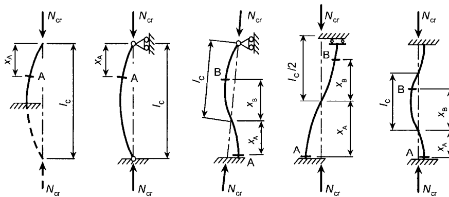
A und B sind Beispiele untersuchter Querschnitte, die mit Querstrichen gekennzeichnet sind. Siehe Tabelle 6.8 zu Knicklängen l_c = kL .
