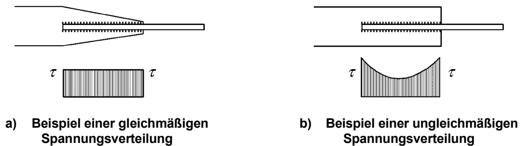
Bild 8.16 — Spannungsverteilungen in Verbindungen mit Kehlnähten A1
