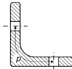
Bild 6.8 — Winkel mit Löchern in beiden Schenkeln
