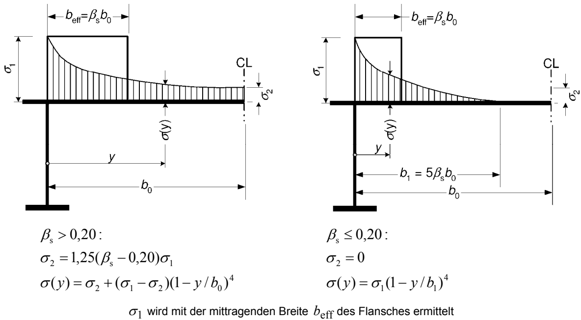
Bild K.3 — Längsspannungsverteilung über die Plattenbreite infolge der Schubverformung
