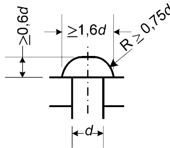
Bild C.1 — Mindestabmessungen des Kopfes von Massivnieten (ohne Ansenkung)
