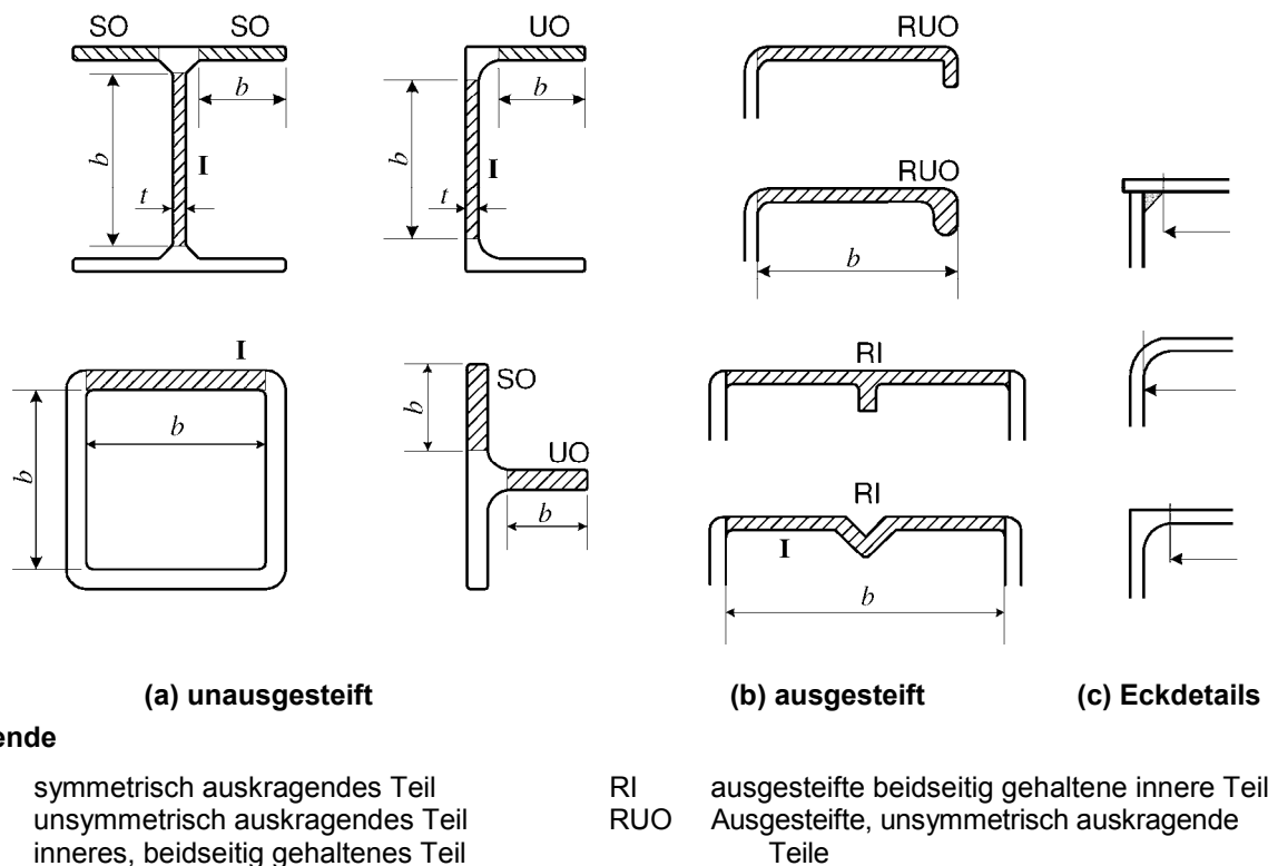
Bild 6.1 — Grundtypen von Querschnittsteilen
