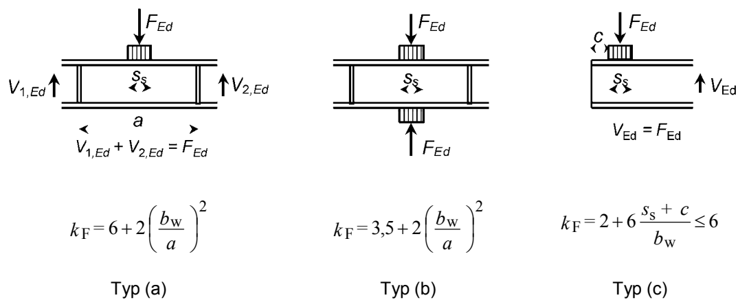
Bild 6.30 — Einleitung von Querlasten und zugehörige Beulwerte
