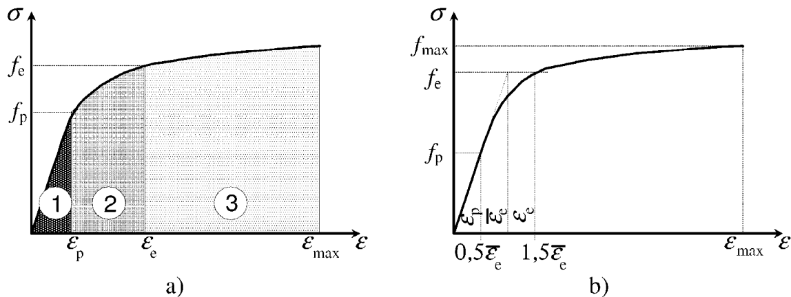
Bild E.3 — Kontinuierliche Modelle der Form \sigma = \sigma(\varepsilon)
