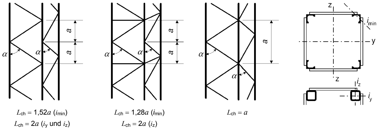
Bild 6.16 — Gitterstützen mit Stäben auf vier Seiten und Knicklänge L_{ch} der Gurtstäbe
