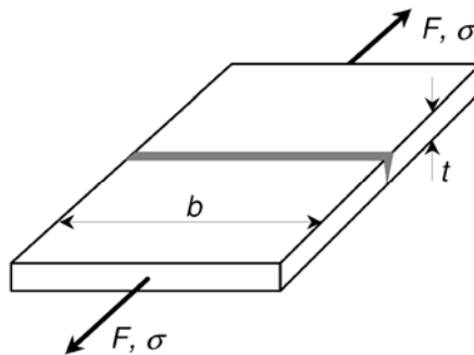
Bild 8.14 — Stumpfnahht mit Normalspannungen
