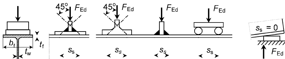
Bild 6.31 — Lasteinleitungslänge
