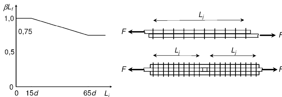
Bild 8.10 — Lange Anschlüsse
