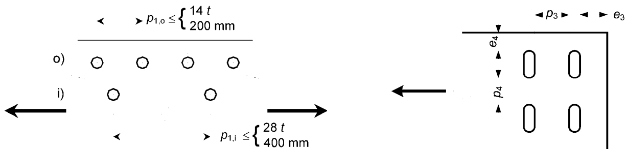
Bild 8.2 — Versetzte Lochanordnung bei druckbeanspruchten Bauteilen
