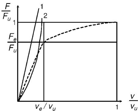
Bild L.3 — Wichtige Verbindungstypen
