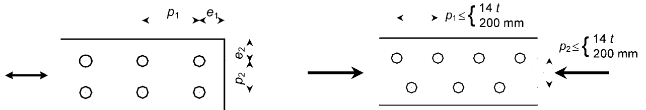
Bild 8.1 — Bezeichnungen der Abstände
