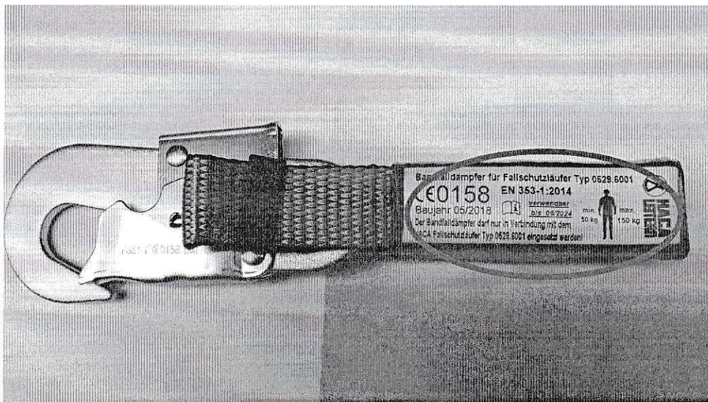
Foto 1: Verwendbar bis Datum eines Bandfalldämpfers
